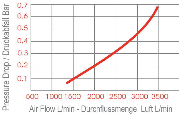
Air 6 Bar
